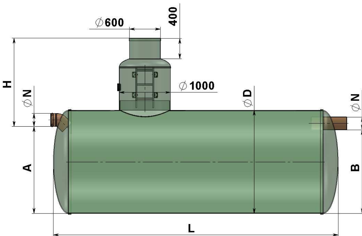
Рисунок 1 – Пескоотделитель «Helyx-ПО»
