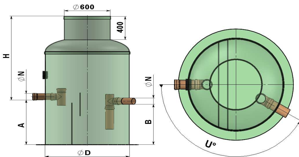
Рисунок 2 – Жиросепаратор вертикального типа
