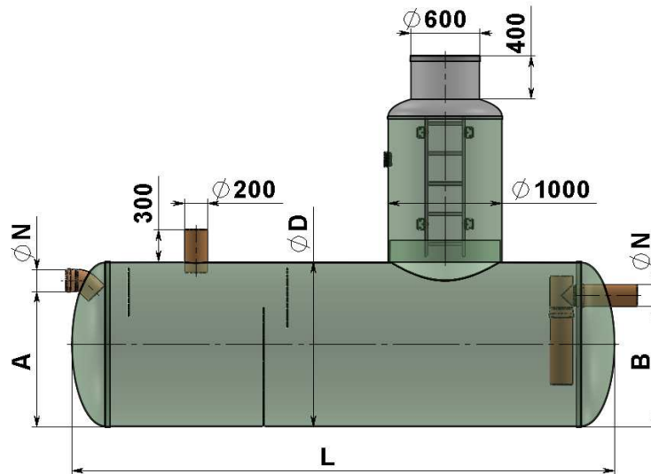
Рисунок 1 – Жиросепаратор горизонтального типа
